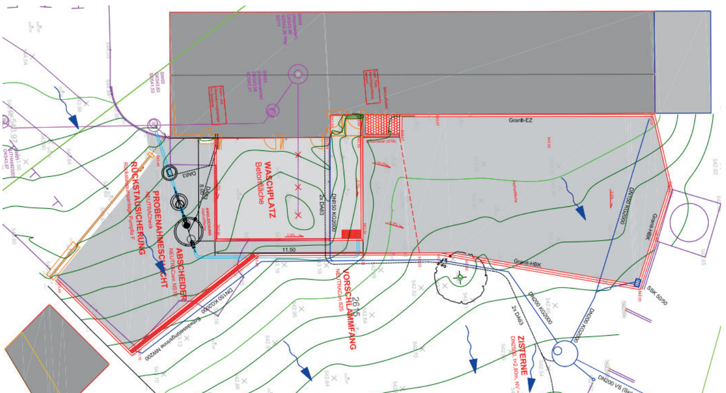
Abb. Bauhof, Neubau Waschplatz. Wolfgang Häusele, Planung im Ingenieurbau
